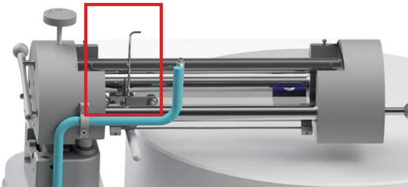
Abb. 19: Befestigen des Headshells (Rückansicht)
