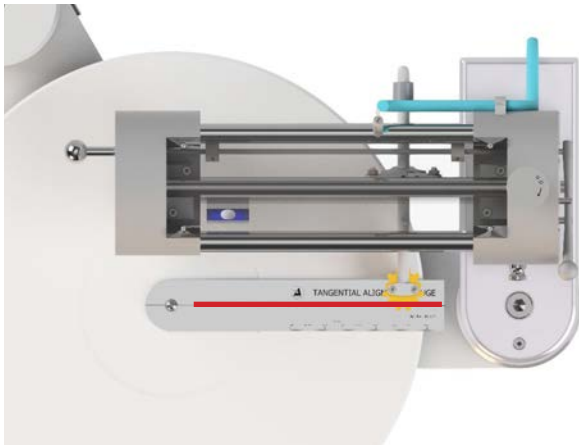
Abb. 26: Einstellung der Tangentialen
