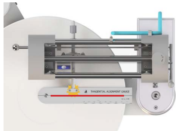
Abb. 26a: Einstellung der Tangentialen
