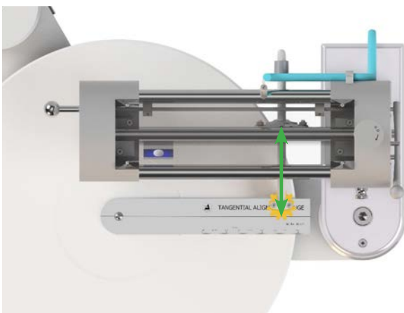
Abb. 24: Abstand zwischen Headshell-Schraube und Diamanten des Tonabnehmers ca. 62 mm
