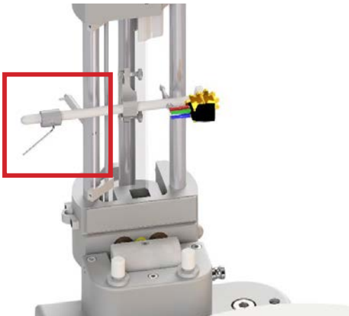
Abb. 21: Befestigen der Gegengewichte
