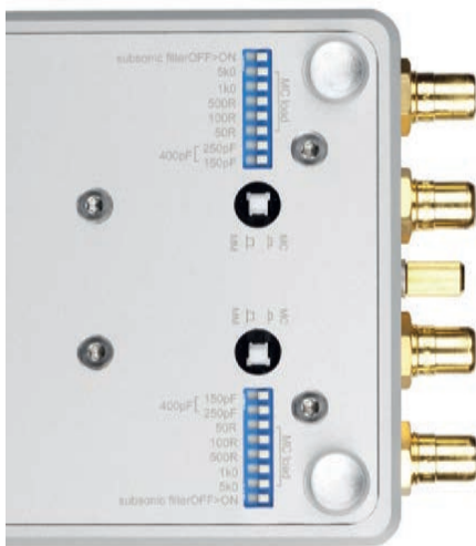
Abb. 2.1: Geräteunterseite
