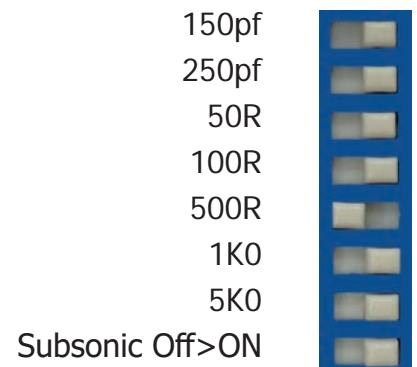
Abb. 2.3: Einstellung 500 Ohm, Subsonic „ON“
