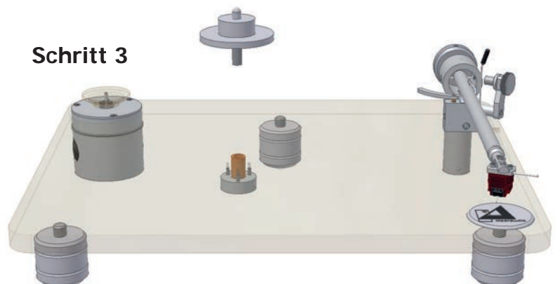
Abb 3: Abnehmen des Standard Lageroberteils
