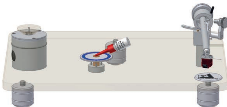
Abb. 9: Synthetisches Lageröl (2-3 Tropfen) in die Lagerbuchse geben.
