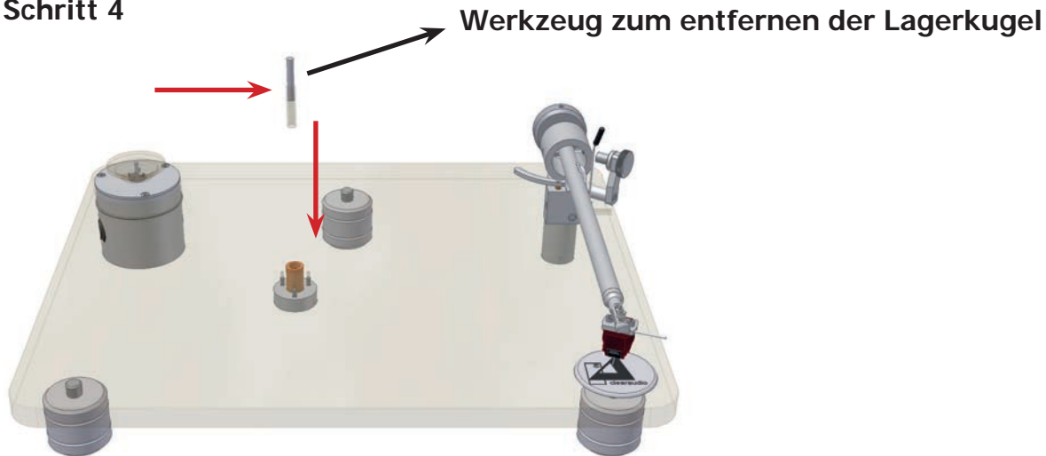
Abb. 4: Entfernen der Lagerkugel: Bitte nehmen Sie die Vorrichtung (im Lieferumfang erhalten) zur Hand.
