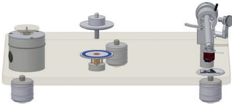
Abb. 10: Aufsetzen des oberen CMB- Lagerteils auf die Achse
