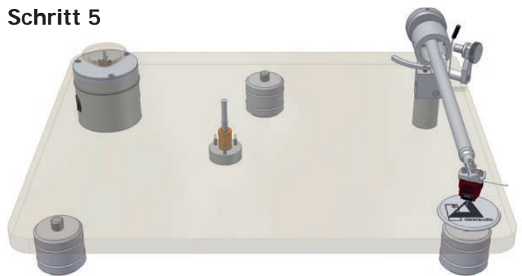
Abb. 5: Entfernen der Lagerkugel: Stecken Sie die Vorrichtung in die Lagerbuchse und üben Sie einen leichten Druck aus.
