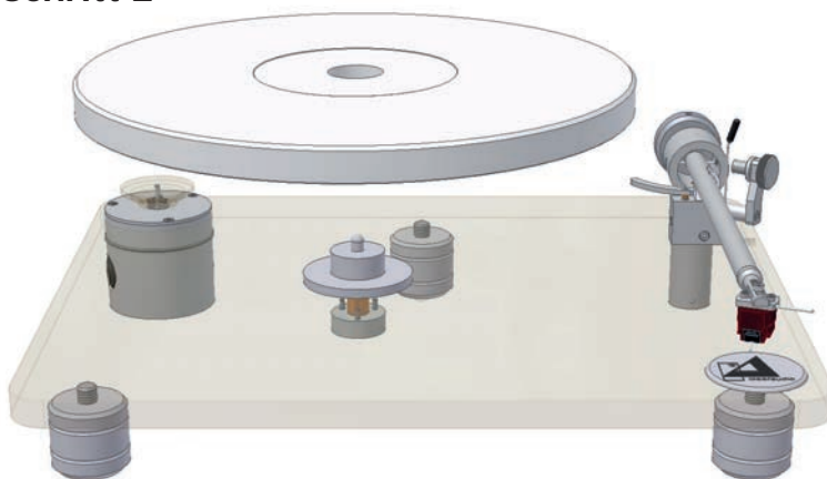
Abb. 2: Abnehmen des Plattentellers
