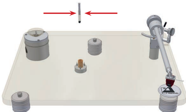
Abb. 6: Entfernen der Lagerkugel: Ziehen Sie die Vorrichtung wieder aus der Lagerbuchse. Nun ist die Lagerkugel entfernt.
