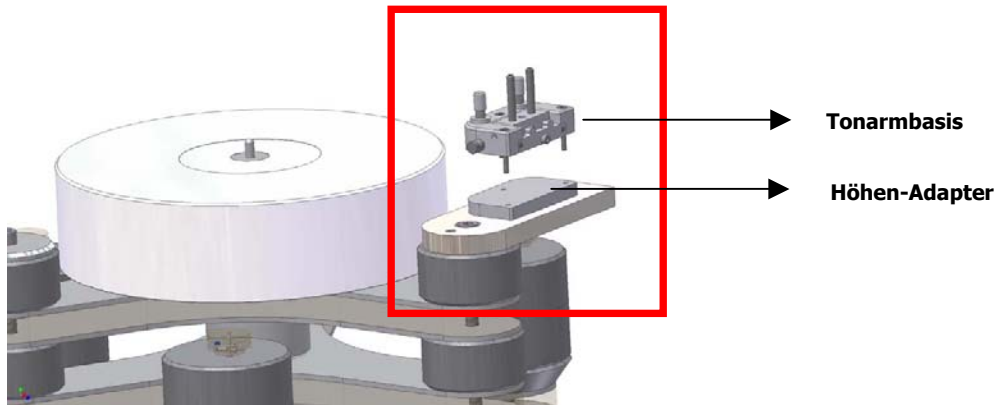
Abb.2: Befestigen der Tonarmbasis
