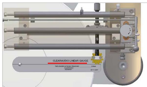
Abb.17: Einstellung der Tangentialen
