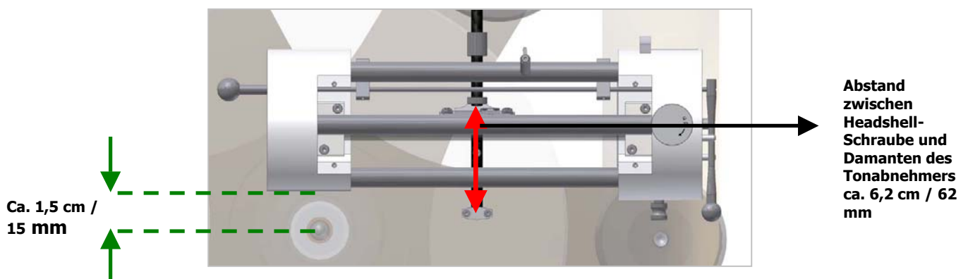
Abb.9: Position nach Einsetzen des Headshells
