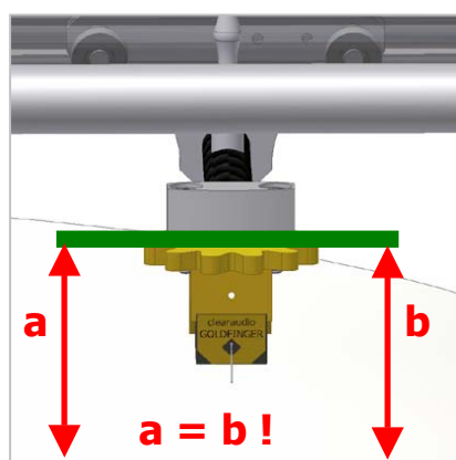
Abb.16: Azimuth - Einstellung
