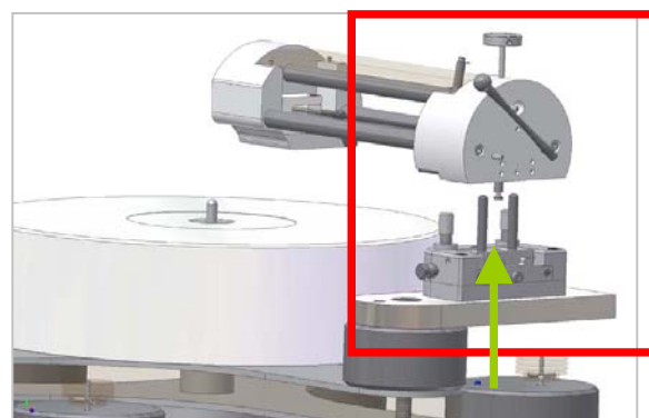
Abb.5: Aufsetzen des Tonarms
