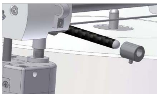
Abb.12: Aufsetzen der Gegengewichte
